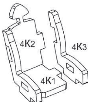
Сборка сидений. Блок К
