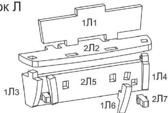
Сборка заднего бампера.
