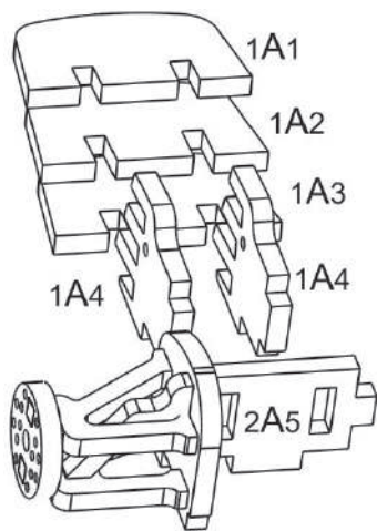
Сборка передней подвески и радиаторной решётки. Блок А
